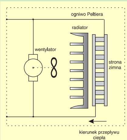
Rys. 2. Schemat ideowy chłodziarki.
